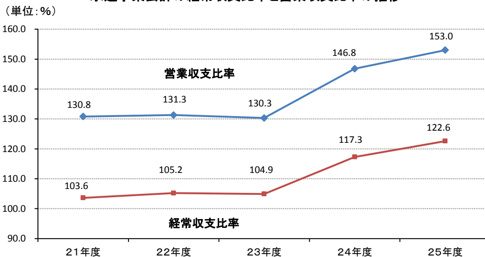
水道事業会計の経常収支比率と営業収支比率の推移
