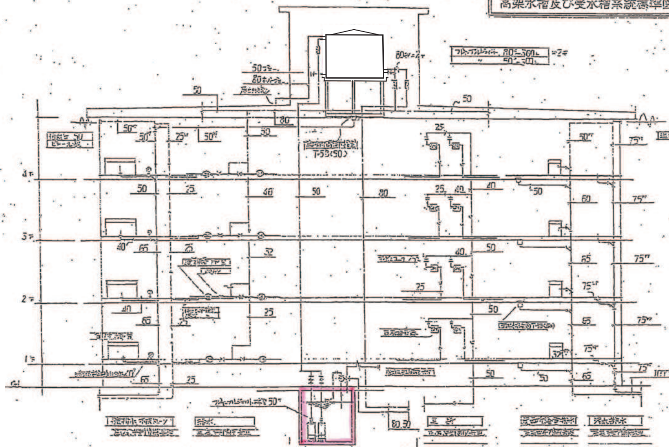
高架水槽及び受水槽系統標準図
