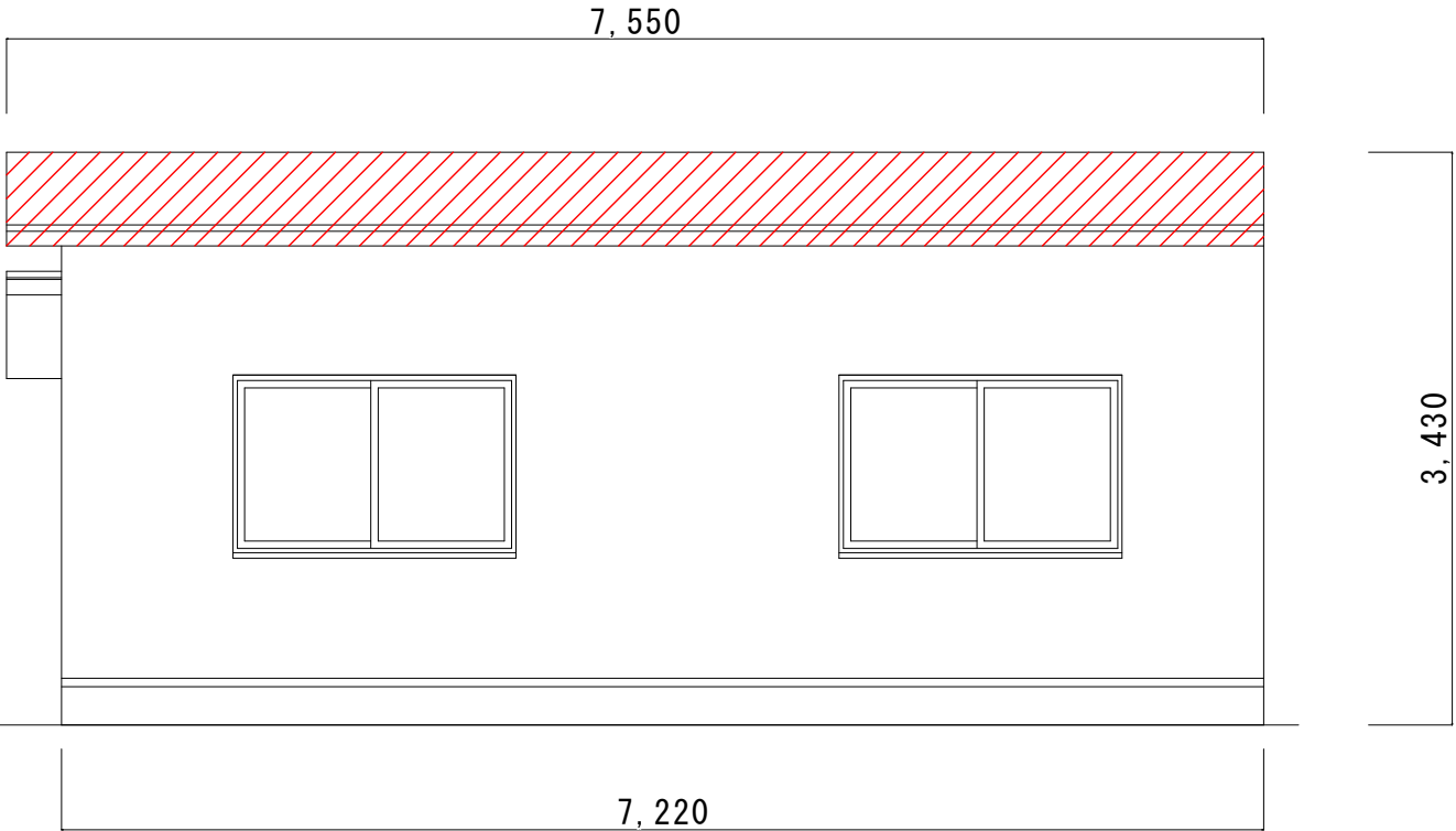
南面立面図
