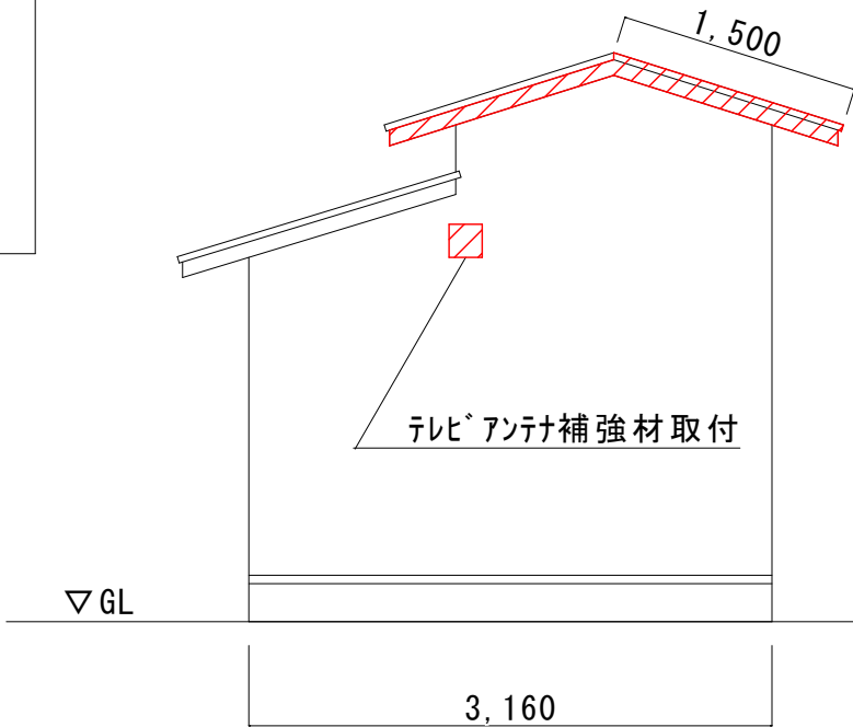
西面立面図
