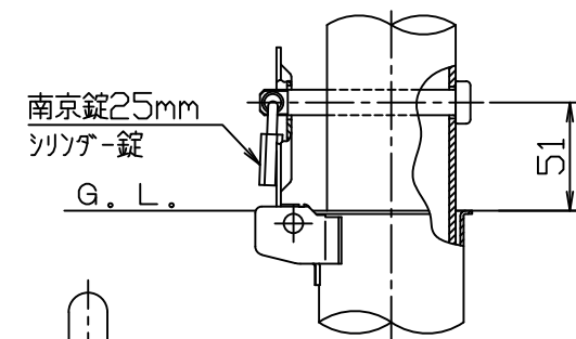
施錠部詳細図
