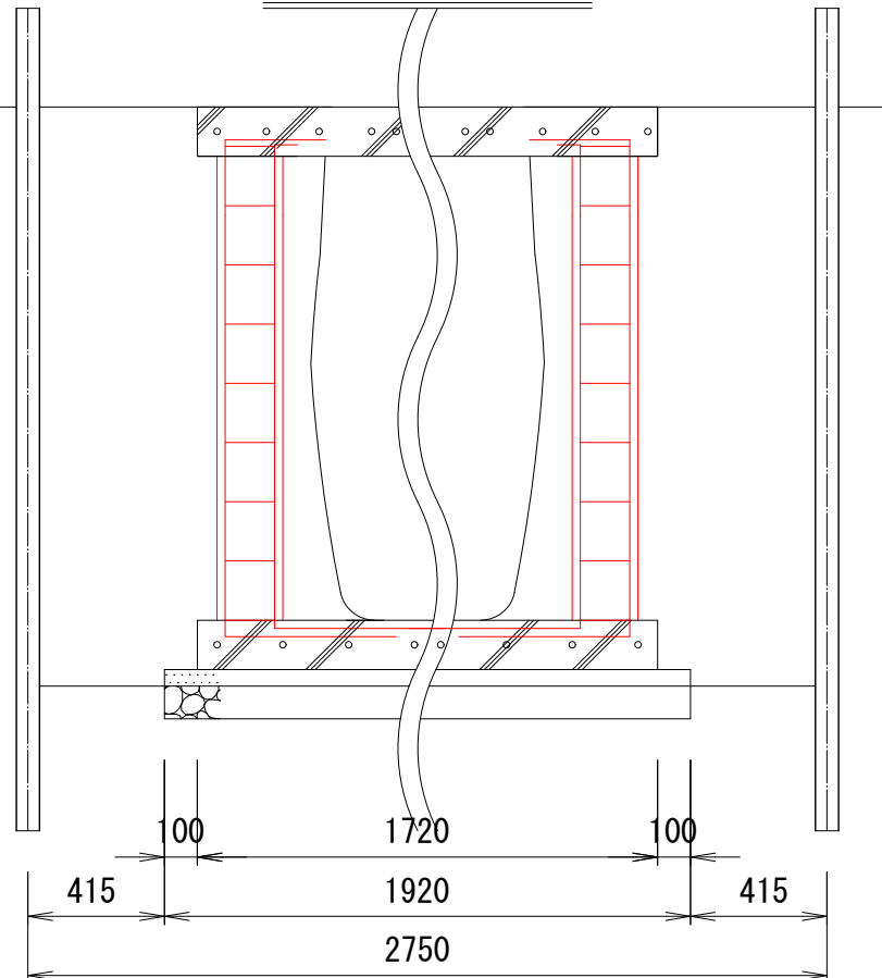
B-B' 断面図
