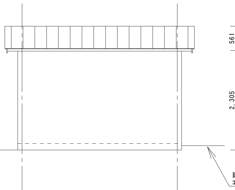
東側立面図 S=1/50
