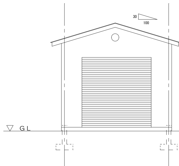
北側立面図 S=1/50
