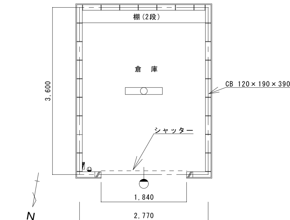
平面図 S=1/50
