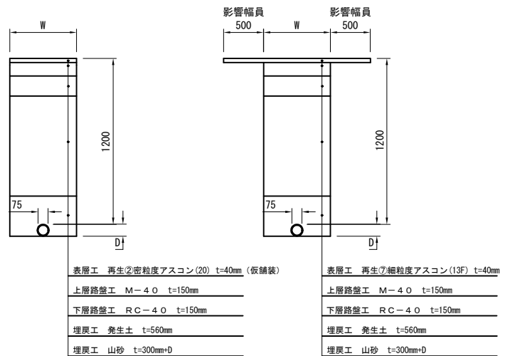
配管標準断面図（市道・車道）
