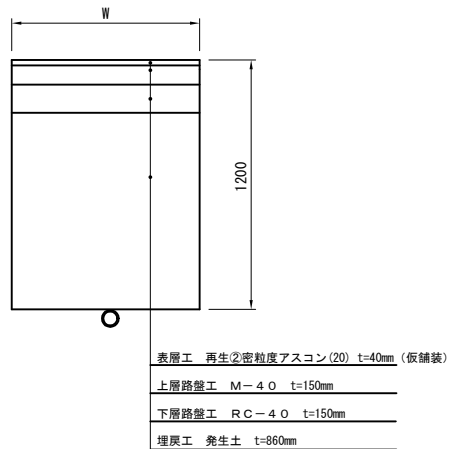
試験掘削標準図（市道・車道）
