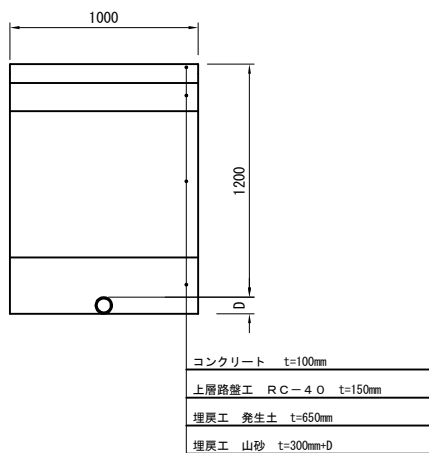
配管標準断面図（コンクリート）
