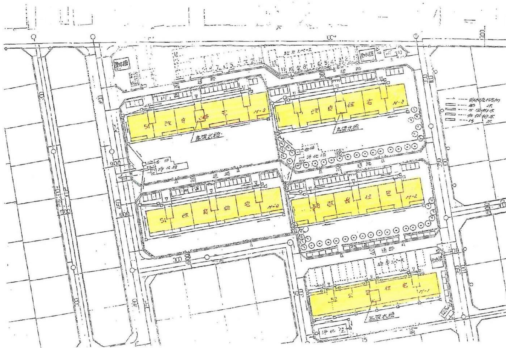
向ヶ丘住宅配置図 S=Free
