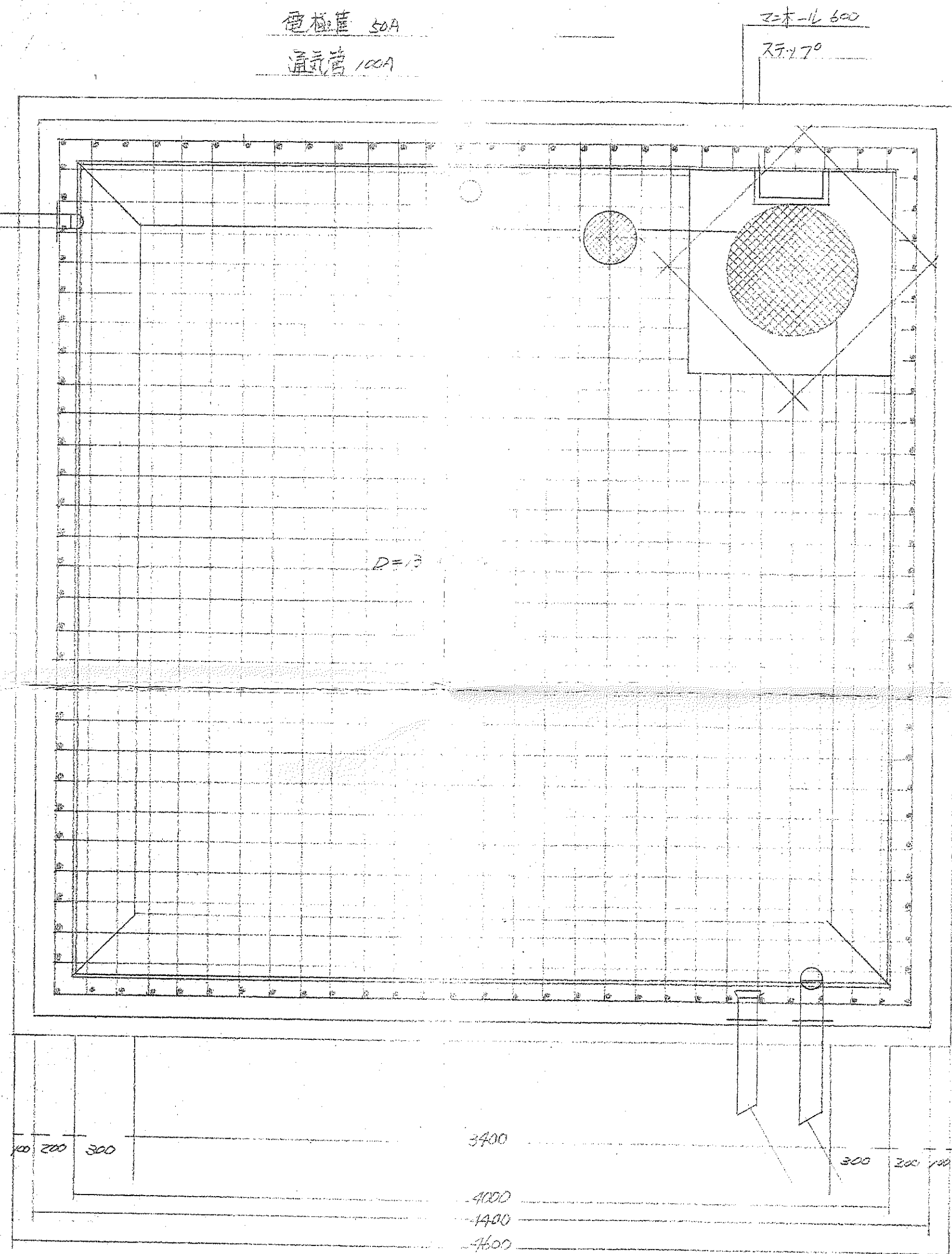
平面圖
