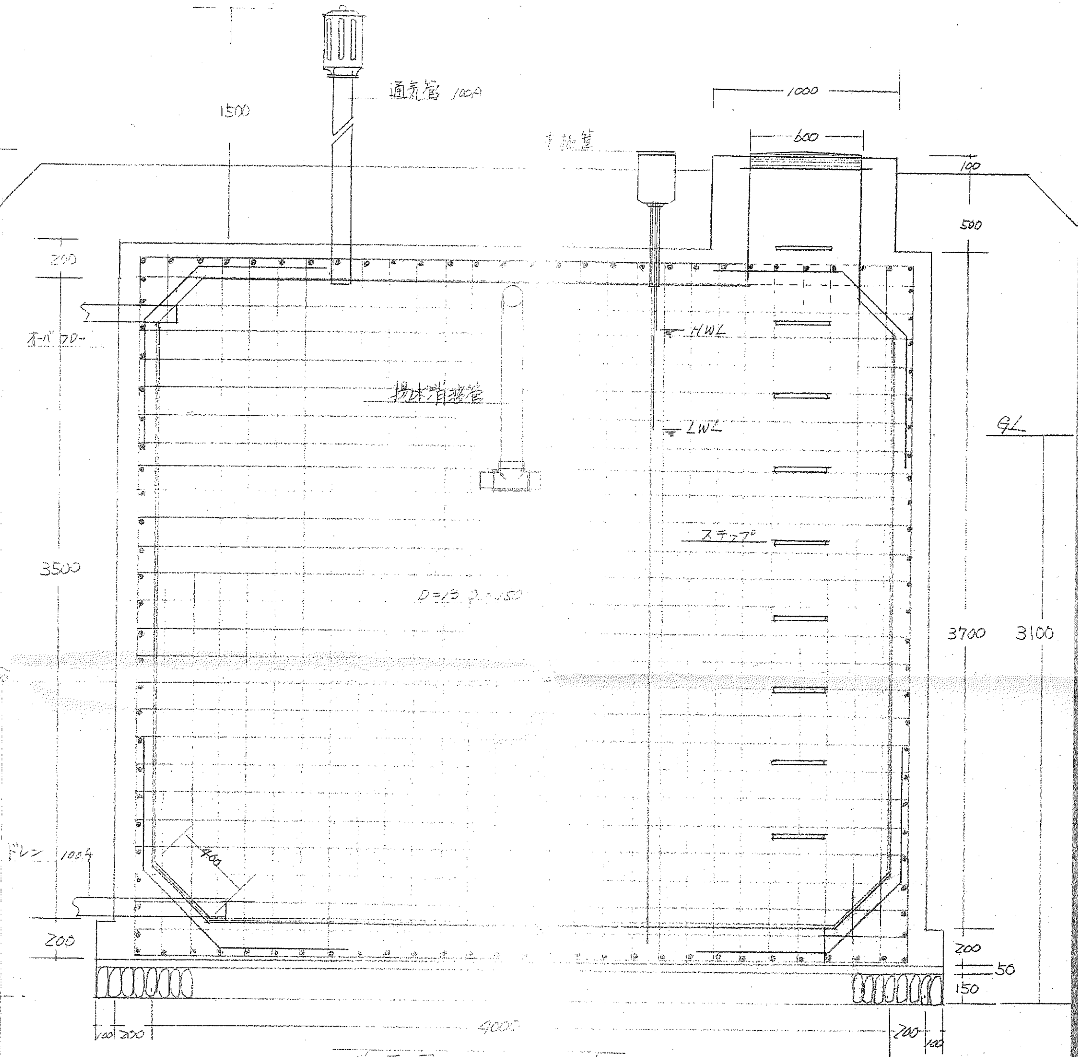
断面圖
