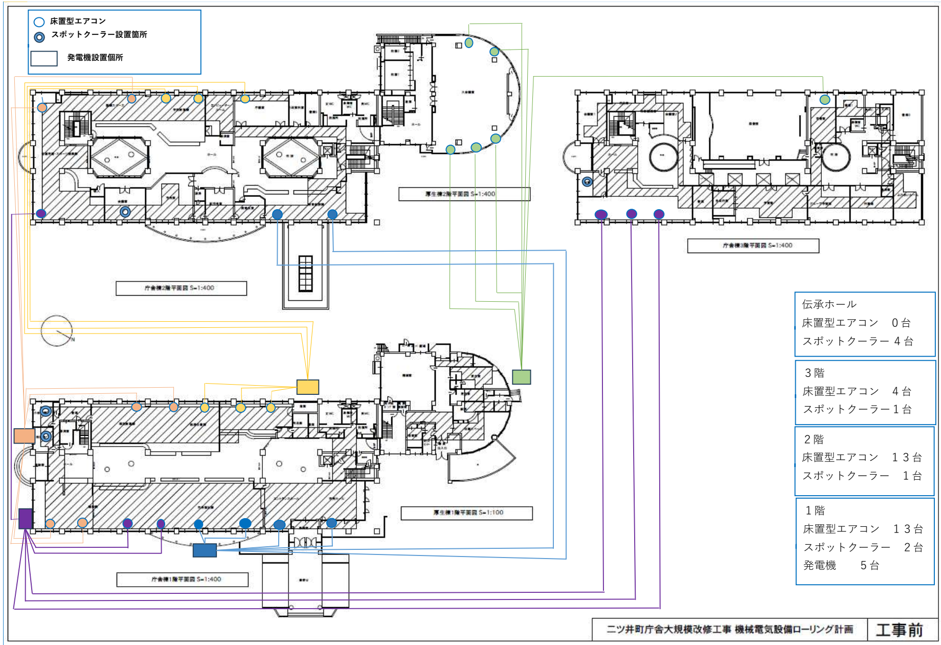
仮設空調機器及び発電機配置図
