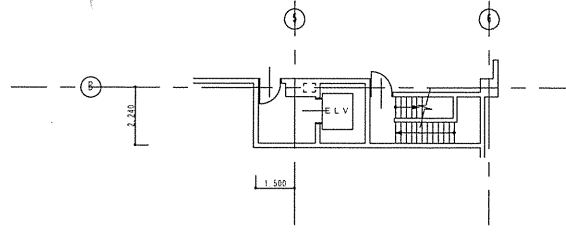
地下中階平面図 S = 1 : 100
