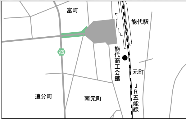
⑥元町1号線(融雪歩道工事) 長さ：90m
