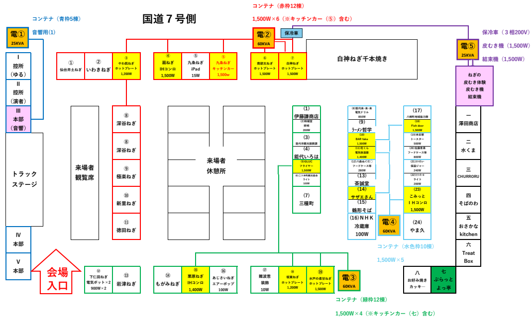
○全国ねぎサミット2026 in のしろ会場仮設電気工事仕様図
